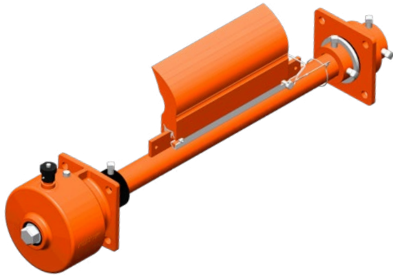
Martin® PV Abstreifer ②
