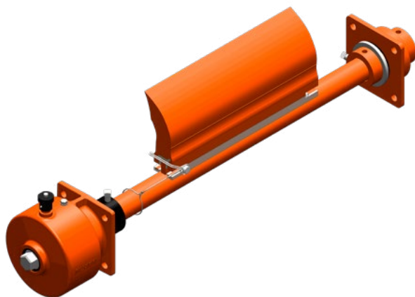
Martin® QC1™ HD Abstreifer ③
