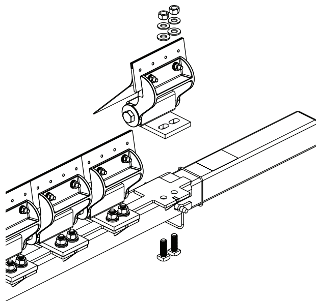
Martin® Orion Estilo Hojas (hardware de montaje incluido en el ensamblaje)
