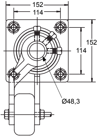
DT2S için Yaylı gergi mekanizması (Ürün no. 37707)
