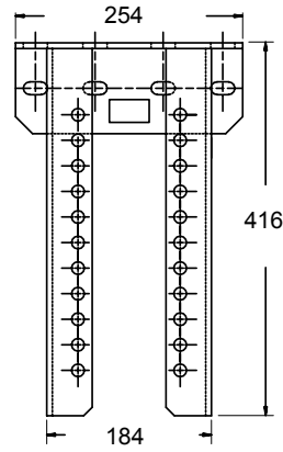
Montaj askısı (Ürün no. 27382+E)
