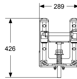
DT2H için Yaylı gergi mekanizması (Ürün no. 37806)
