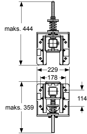
Çift yönlü uygulamalar için yaylı gergi mekanizması (Ürün no. 33599-M)
