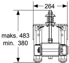
DT2S için Yaylı gergi mekanizması (Ürün no. 37707)
