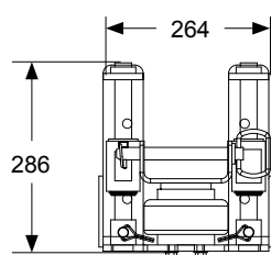
DT2S için Havalı gergi mekanizması (Ürün no. 37707-A)
