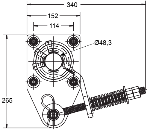
Kauçuk körüklü havalı gergi mekanizması (Ürün no. 32745+E)
