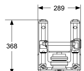
DT2H için Havalı gergi mekanizması (Ürün no. 37806-A)
