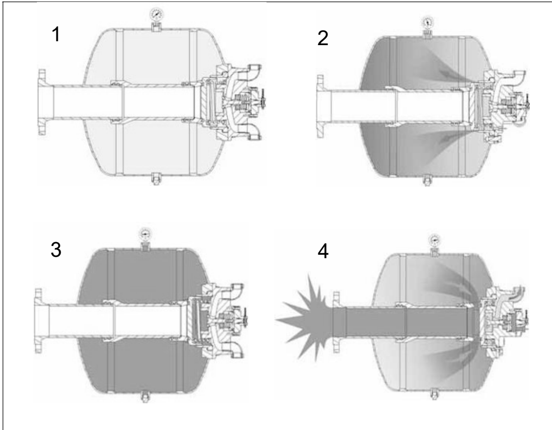
Şekil 1: Hava Şoku dolum ve tahliyesi
