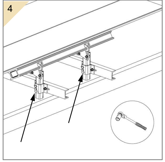
Yüksekliğin ayarlanması
