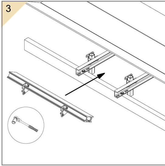
Barların montajı
